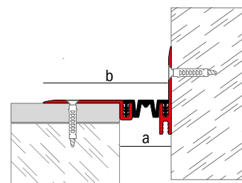
a: 24, 34 y 44 mm. | b: 72, 82 y 92 mm. length: 2,5 m.
