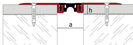
a: 24, 34 y 44 mm. | h: 11 mm. length: 2,5 m.
