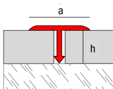
a: 15 mm. | h: 7 mm. length: 2,5 m.
